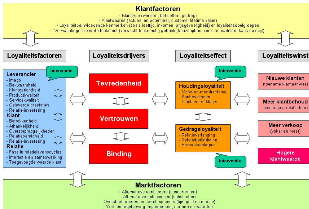
Figuur 1: KlantLoyaliteitModel ©
